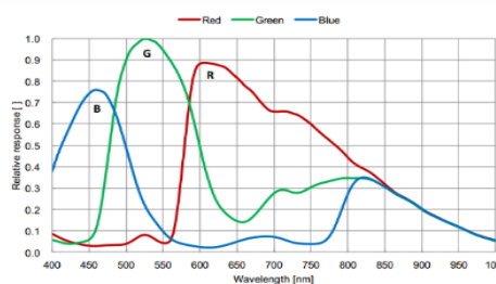
MV-CA023-10GC 量子效率
