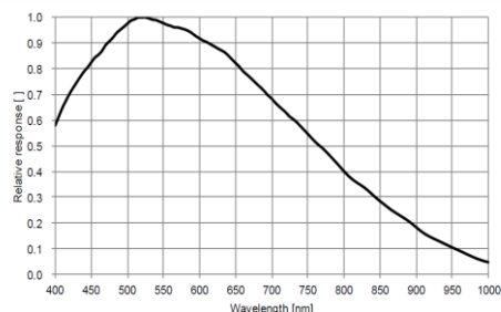
MV-CA023-10GM 量子效率
